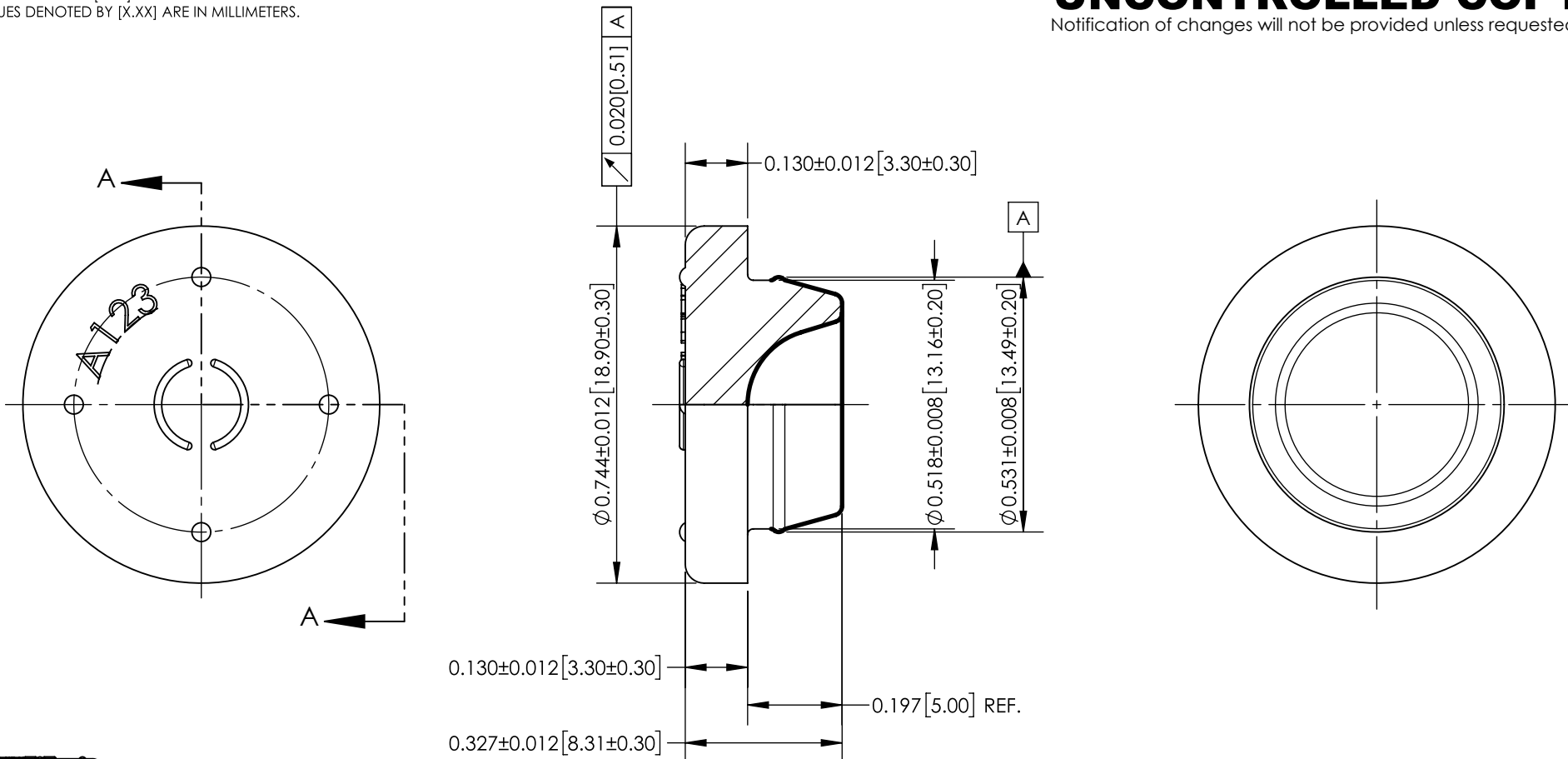
SECTION A-A
